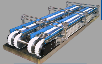
Zahnriemenband
