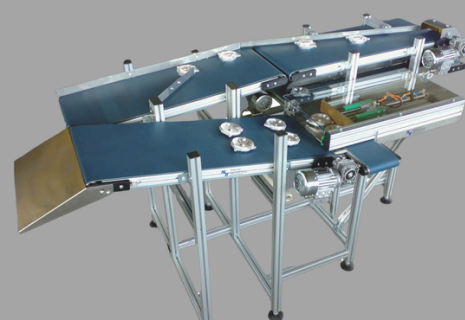
Wendezuführanlage
