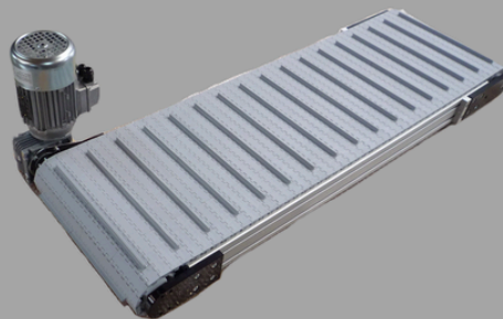
Scharnierplattenband
